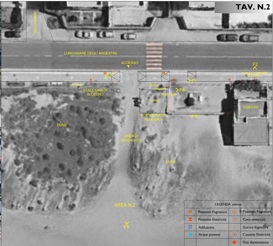
PLANIMETRIA DELL'AREA
